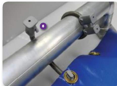
6 130133 StormFix spanner grijs 180 mm StormFix stretcher grey 180 mm StormFix Spanngummi Grau 180 mm
