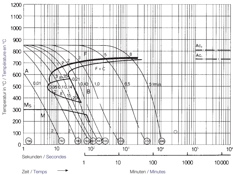
Diagramme TTT refroidissement continu
