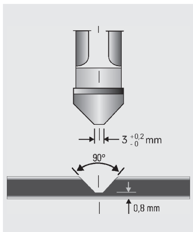
Fraise à disque pour rainures en V de 90°
