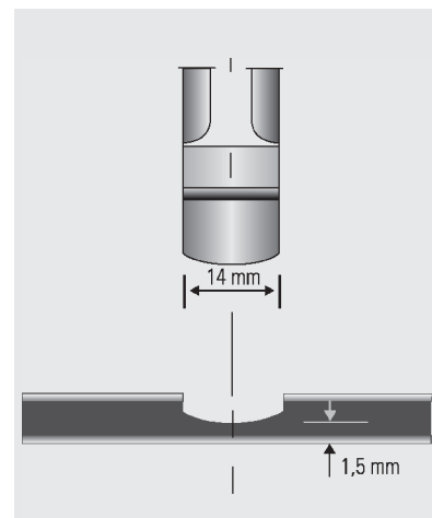
Fraise à disque pour rainures rectangulaires
