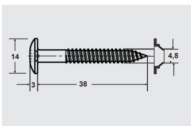
Vis de façade à tête goutte-de-suiif
