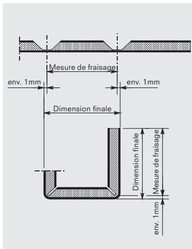
Détermination de la mesure de fraisage
