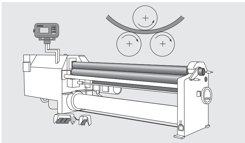
Cintrage sur cintreuse à rouleaux
