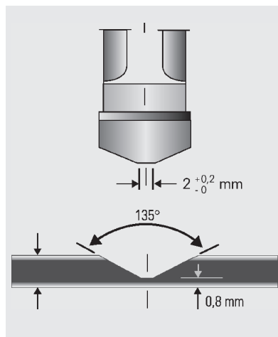
Fraise à disque pour rainures en V de 135°
