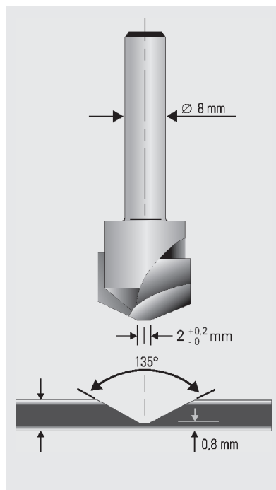
Fraises pour rainures en V de 135° MC-fraise N° 491 443 (Festool) MC-fraise N° FV09.01.135 (GIS) MC-fraise N° 79 804 (KWO)
