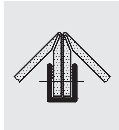
Jointure des plisges, 30mm, profilé 24 569
