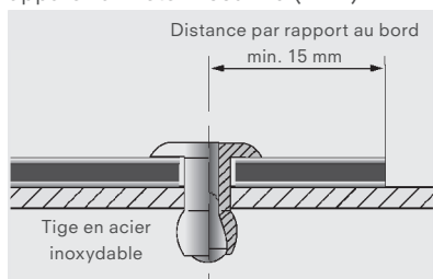
Rivet aveugle à tête plate
