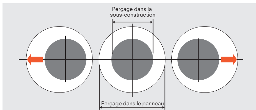
Perçage central
