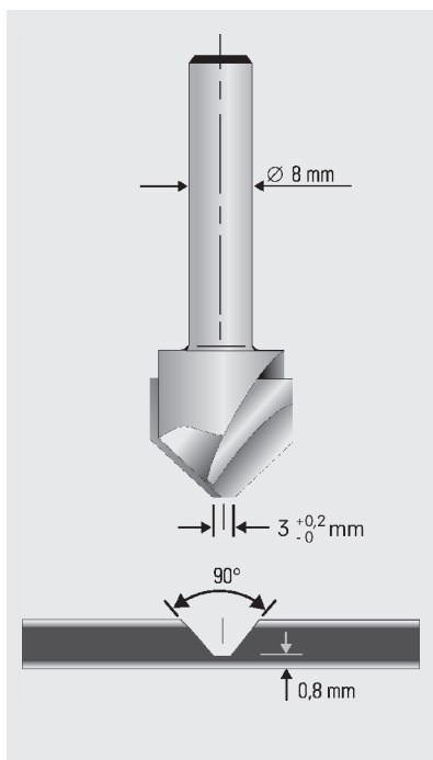
Fraises pour rainures en V de 90° MC-fraise N° 491 444 (Festool) MC-fraise N° FV09.01.090 (GIS) MC-fraise N° 79 803 (KWO)
