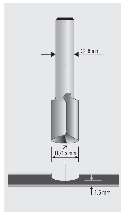
Fraises pour rainures rectangulaires AR-fraise Ø 10 mm N° 79800(KWO) AR-fraise Ø 15 mm N° 79801(KWO)
