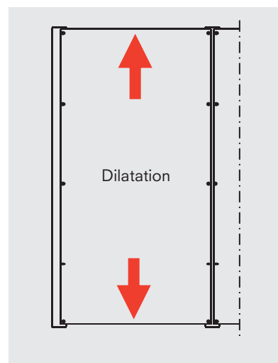
Dilatation dans le sens du profilé support pour sous-construction aluminium, selon avis technique Facteur 0,1 (différence de température 10°C).
