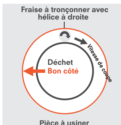
Panneau = pièce à usiner, vitesse de coupe dans le sens des aiguilles d'une montre
