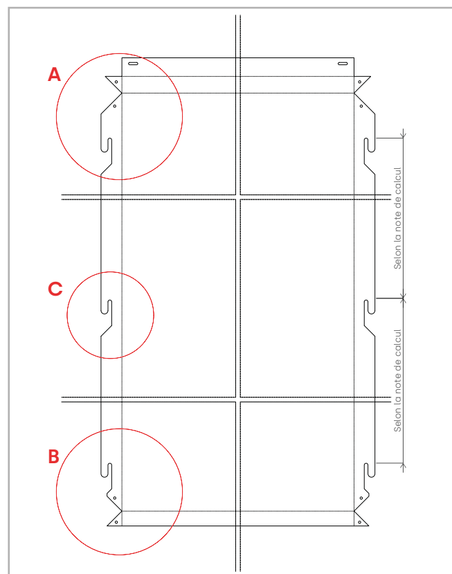
CASSETTE DÉVELOPPÉE
