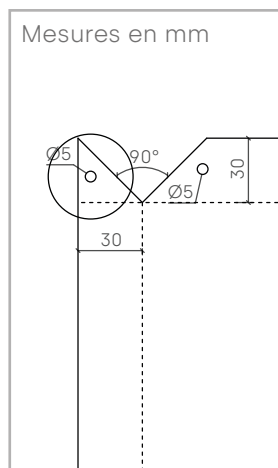
DÉTAIL A
