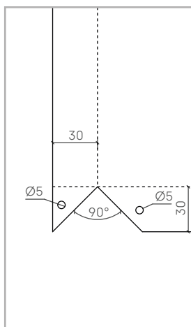
DÉTAIL B
