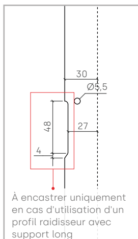
DÉTAIL C
