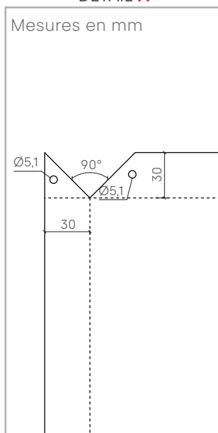
DÉTAIL A
