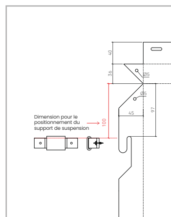
DÉTAIL A
