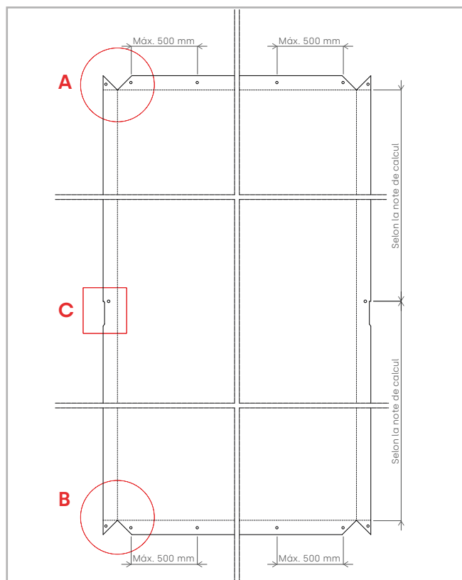
CASSETTE DÉVELOPPÉE
