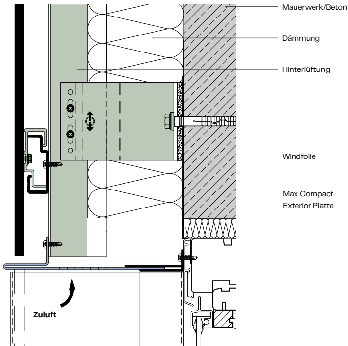
Fenstersturz A101
