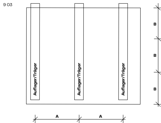
9 03 Abstände Unterkonstruktion
