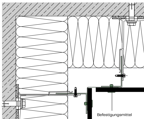
Innenecke A106
