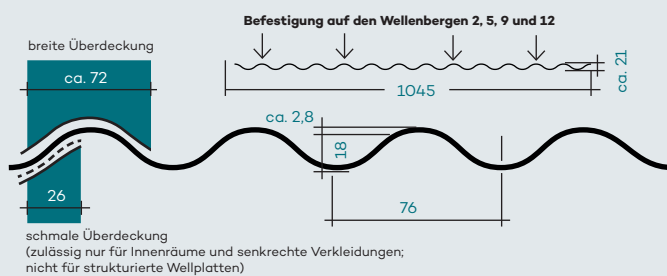
Querschnitt der PLEXIGLAS® Heatstop Cool Blue WP 76/18/2,8
