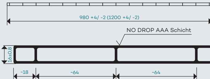
Querschnitt der PLEXIGLAS® Heatstop Cool Blue AAA SDP 16-64 (Maße in mm)
