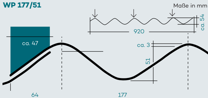
Querschnitt der PLEXIGLAS® Resist WP 177/51 (Maße in mm)
