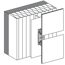
EASY FIX 135° / 135° für vertikale / horizontale Fassadengliederung
