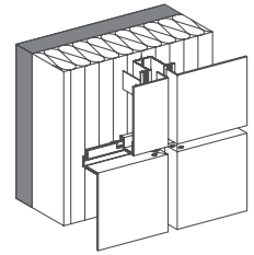
KASSETTE SZ 20 Nut- und Federprinzip für horizontale Fassadengliederung
