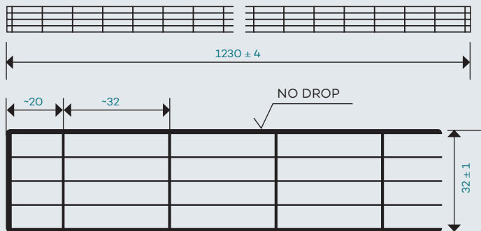
Querschnitt der PLEXIGLAS® Heatstop Cool Blue S5P 32 (Maße in mm)
