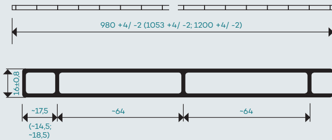
Querschnitt der PLEXIGLAS® Alltop SDP 16/64, schlagzäh-modifiziert (Maße in mm)
