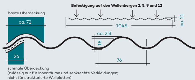
Querschnitt der PLEXIGLAS® proTerra WP 76/18/2,8
